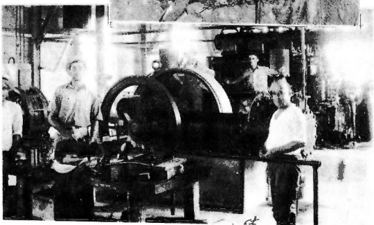
Vista del compresor No. 1 y parte del taller de reparaciones.
